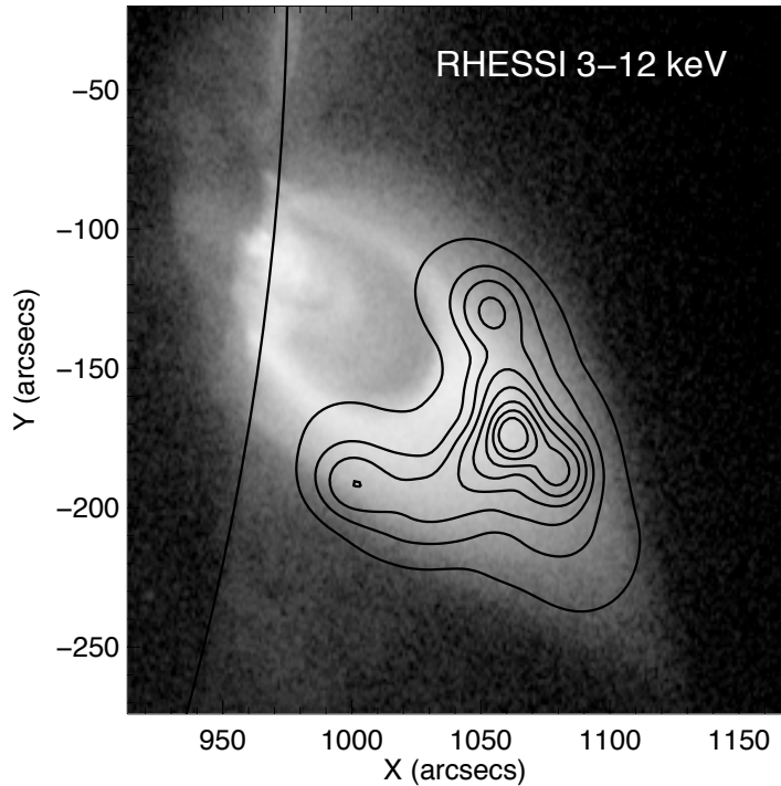
XRT C_poly 17-Dec-2006 20:01:07.456 UT
